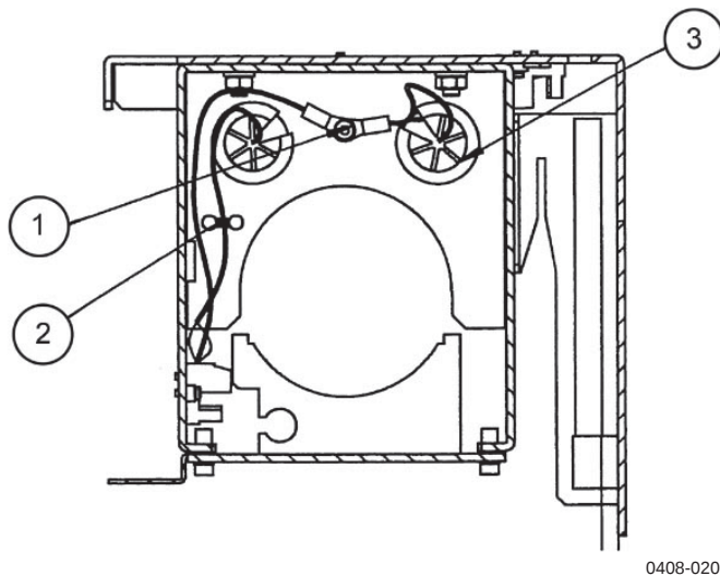
Рисунок 20 Провода заземления внутренней кабельной проводки (вид сверху)
