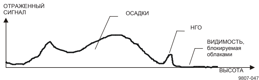
Рисунок 16 Типичный сигнал измерения
