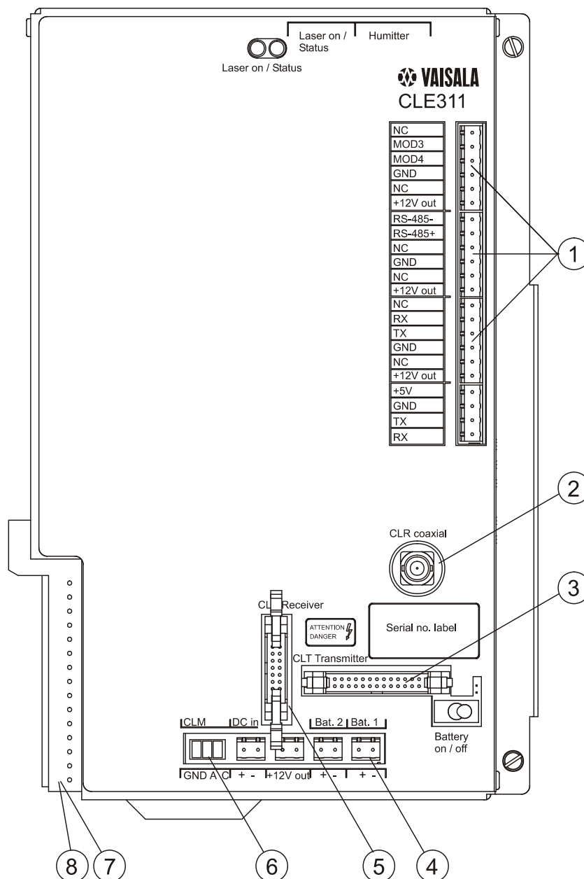
Рисунок 11 Внутренние соединения
