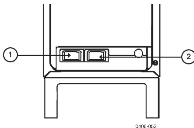
Рисунок 12 Выключатели CL31
