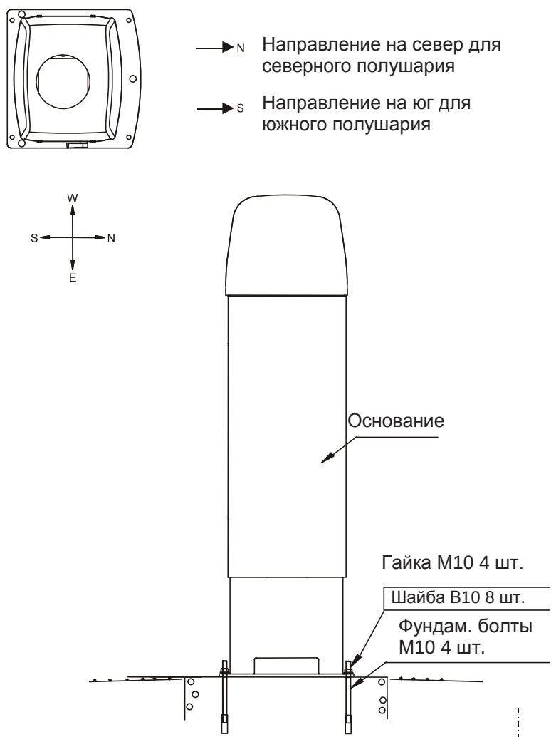
Рисунок 6 Установка экрана
