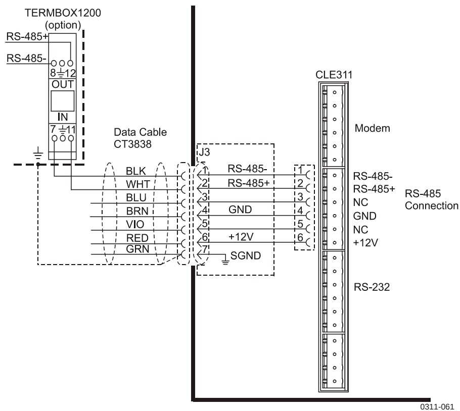
Рисунок 9 Подключение линии связи RS-485
