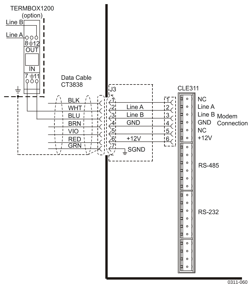
Рисунок 8 Подключение модема для связи
