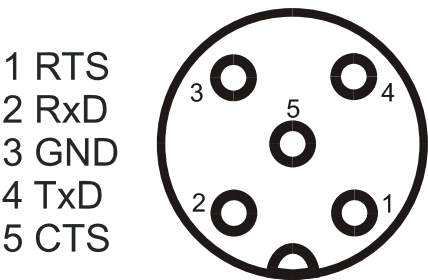
Рисунок 25 Штырьковые соединения разъема J4
