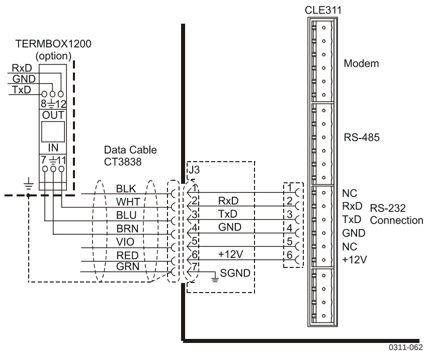
Рисунок 10 Подключение линии связи RS-232
