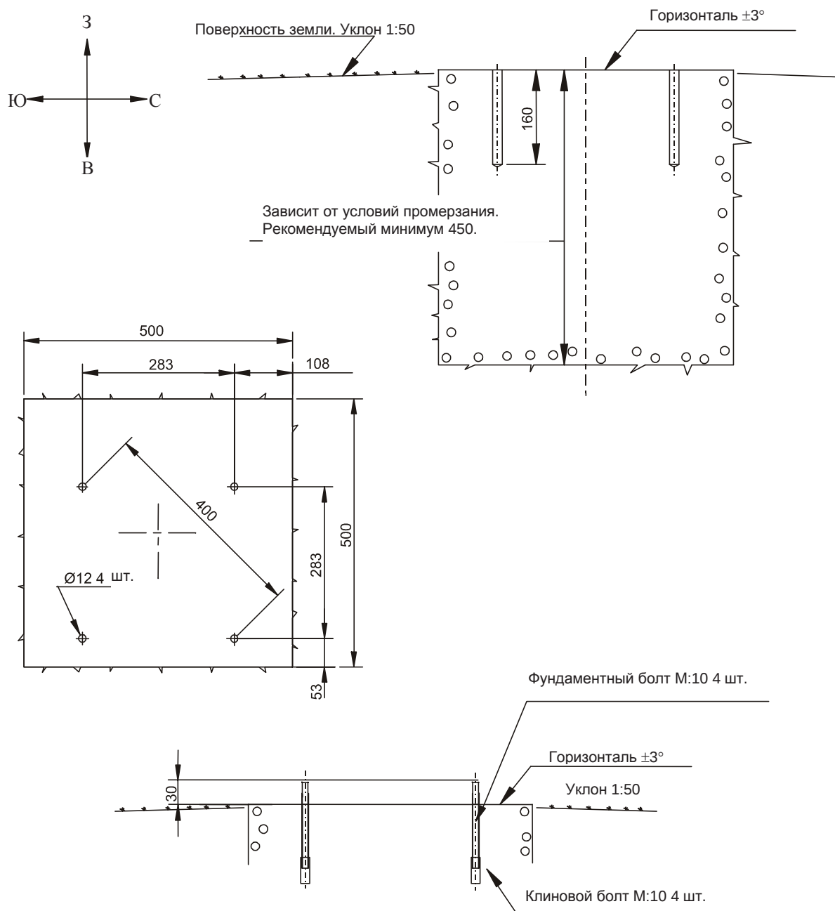
Рисунок 4 Конструкция фундамента
