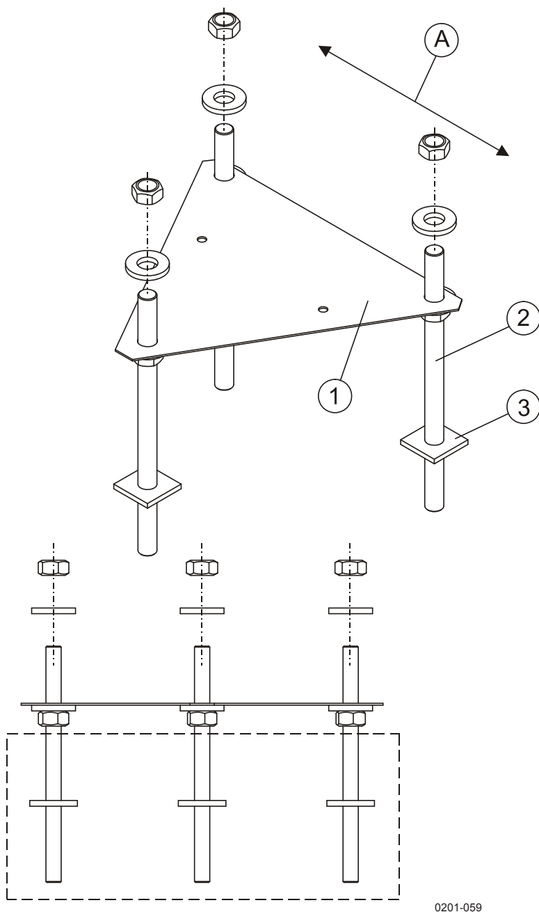
Рис. 6. Возведение фундамента для FS11P
