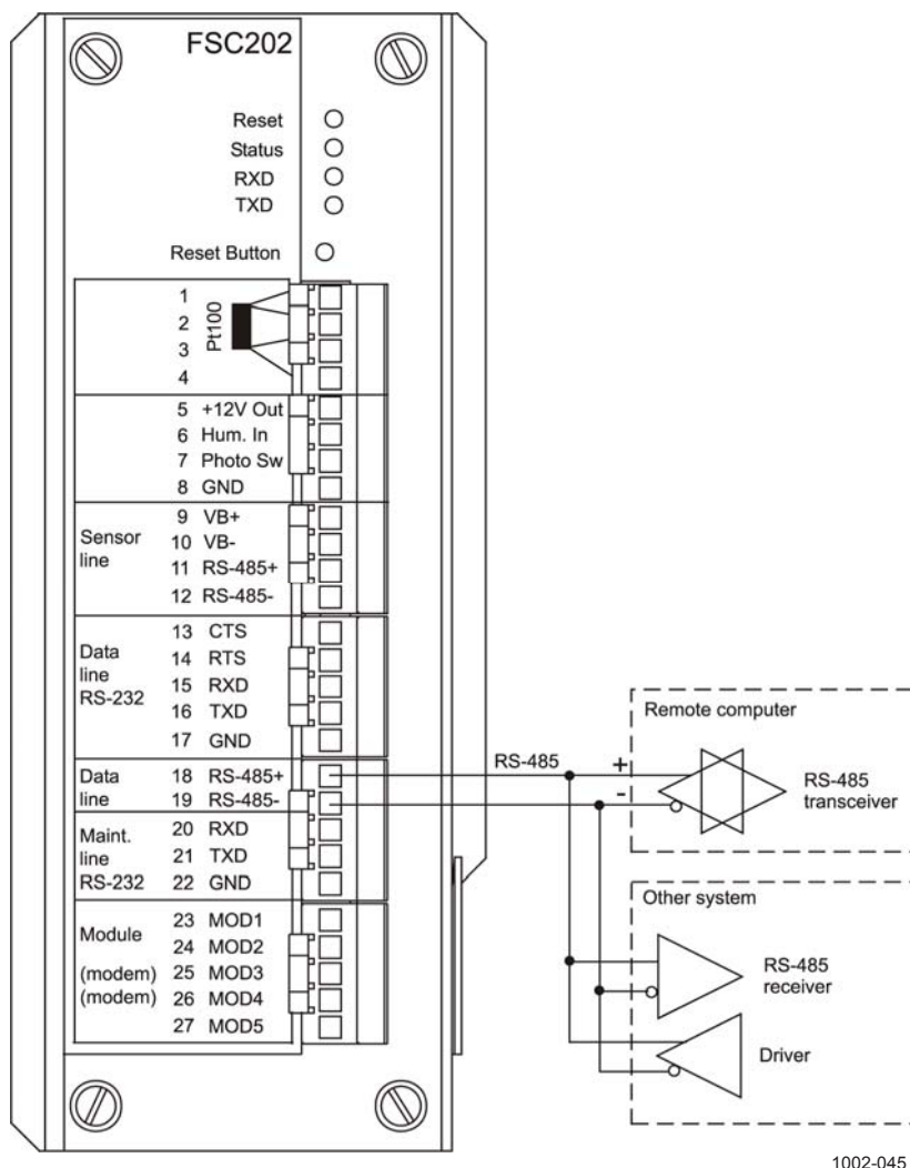
Рис. 27. Связь в стандарте RS-485
