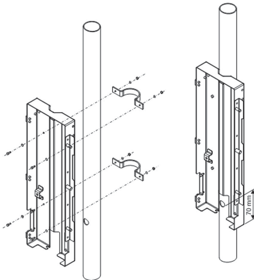
Рис. 12. Монтаж задней панели радиационного экрана
