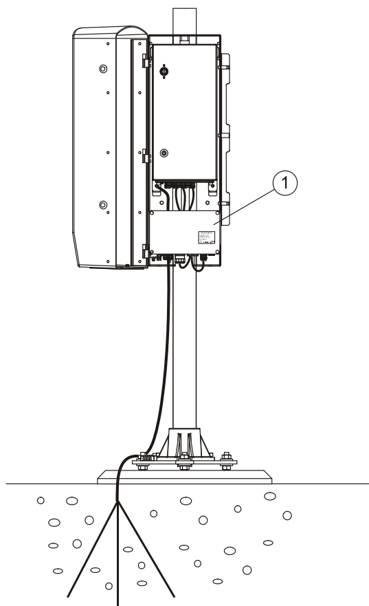
Рис. 4. Распределительная коробка
