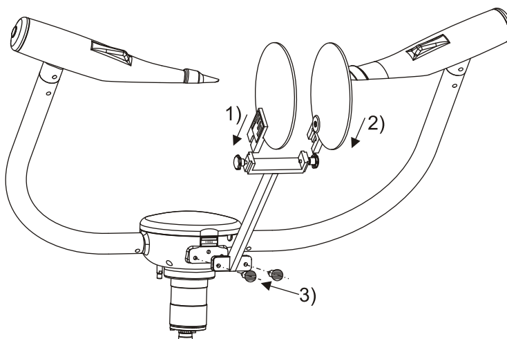
Рис. 41. Сборка и установка калибратора
