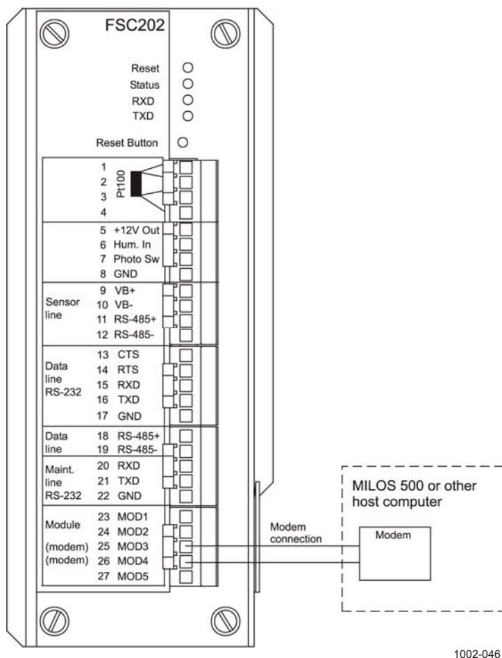
Рис. 29. Подключение модемного кабеля
