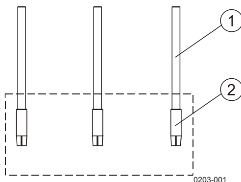
Рис. 7. Монтаж FS11P на существующей поверхности
