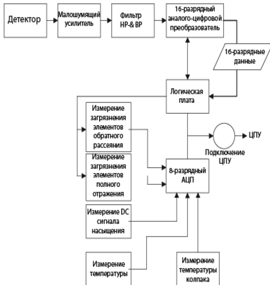
Рис. 38. Блок-схема приемника FSR102
