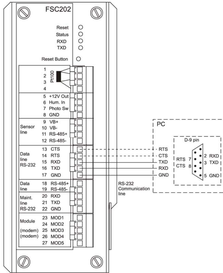
Рис. 26. Вариант связи по протоколу RS-232
