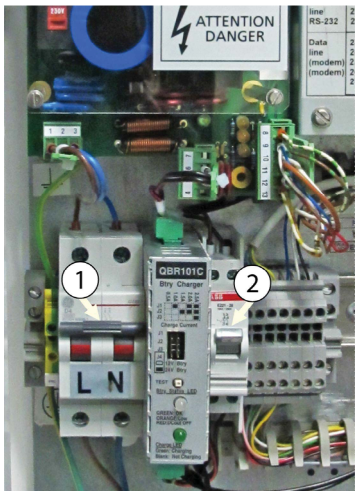
Рис. 34. Включение блока
