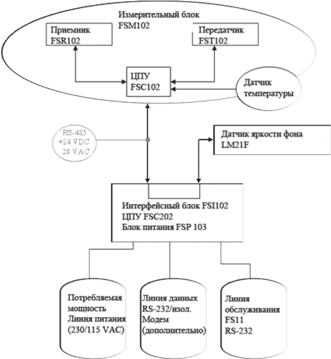
Рис. 35. Блок-схема измерения видимости датчика текущей погоды FS11P
