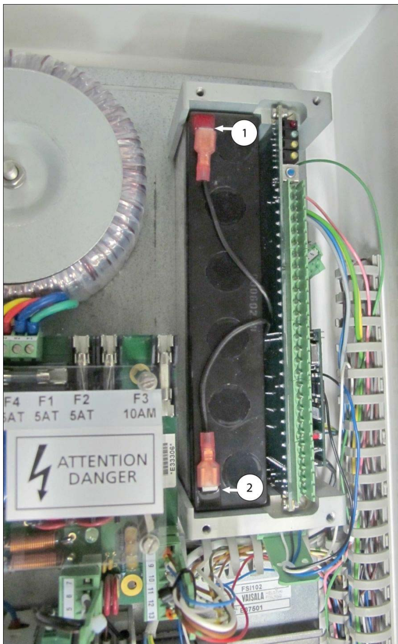
Рис. 22. Резервная батарея без крышки
