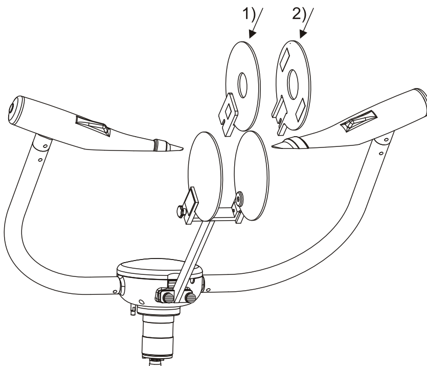
Рис. 42. Установка шаблонных пластин на матовые стекла
