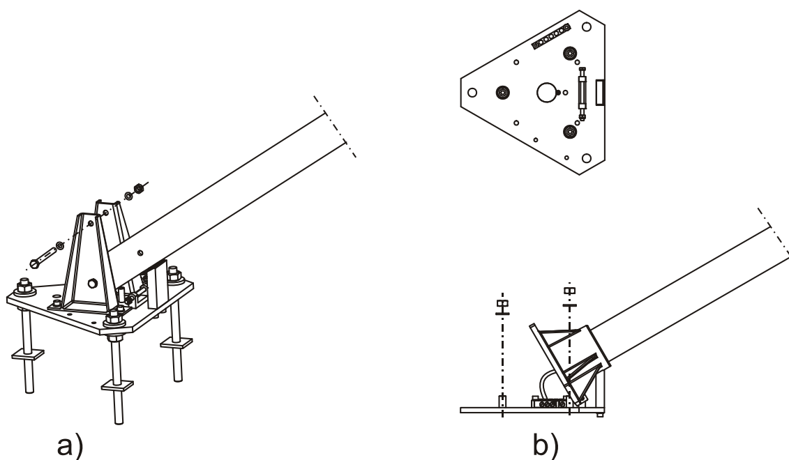
Рис. 13. Наклон алюминиевой и хрупкой мачт
