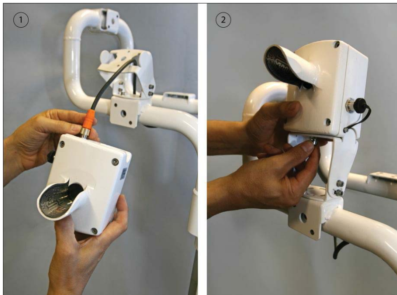
Рис. 18. Монтаж LM21
