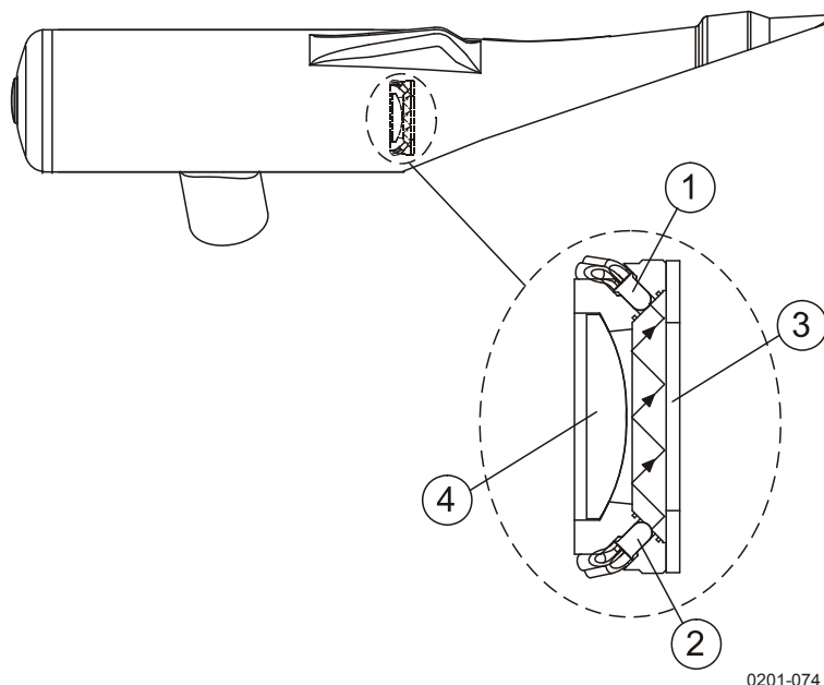
Рис. 37. Принцип измерения загрязненности окна передатчика и приемника FSM102
