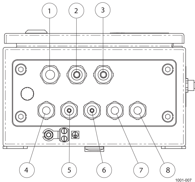
Рис. 23. Кабель корпуса интерфейсного блока
