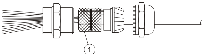
Рис. 25. Инструкция по заземлению кабеля
