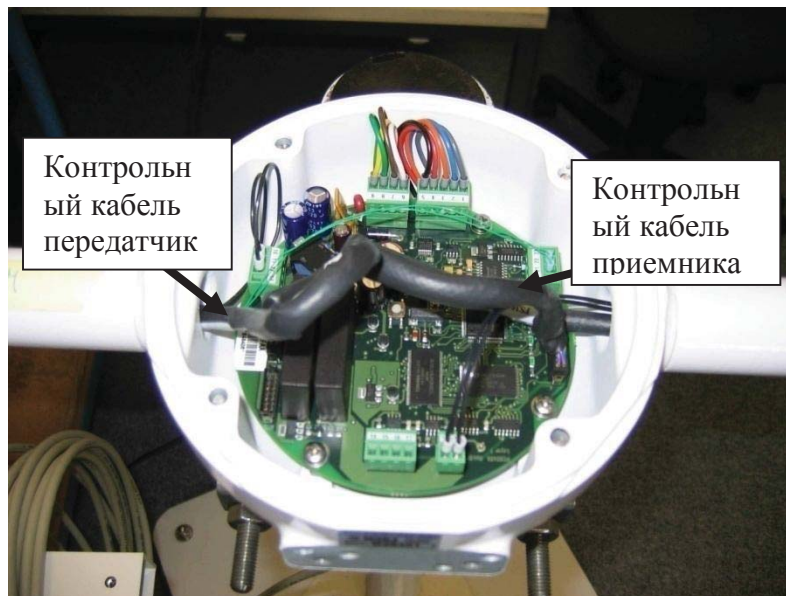
Рис. 43. Контрольные кабели передатчика и приемника датчика текущей погоды
