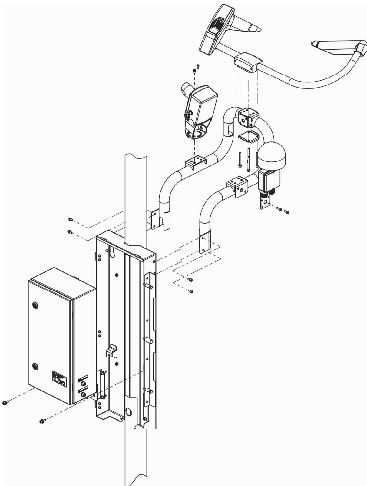
Рис. 20. Монтаж FS11P
