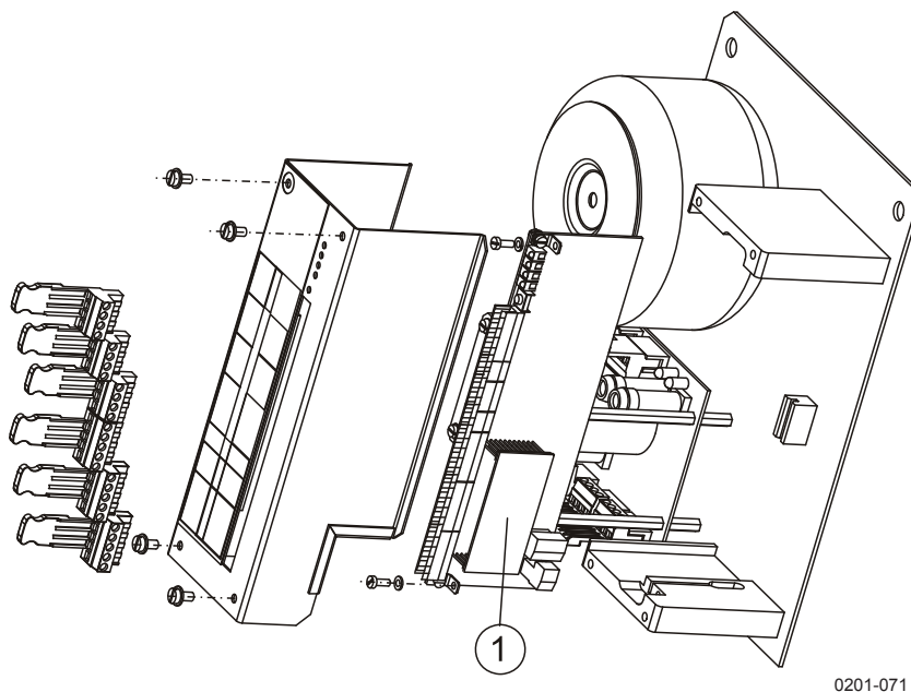
Рис. 30. Установка модема DMX501
