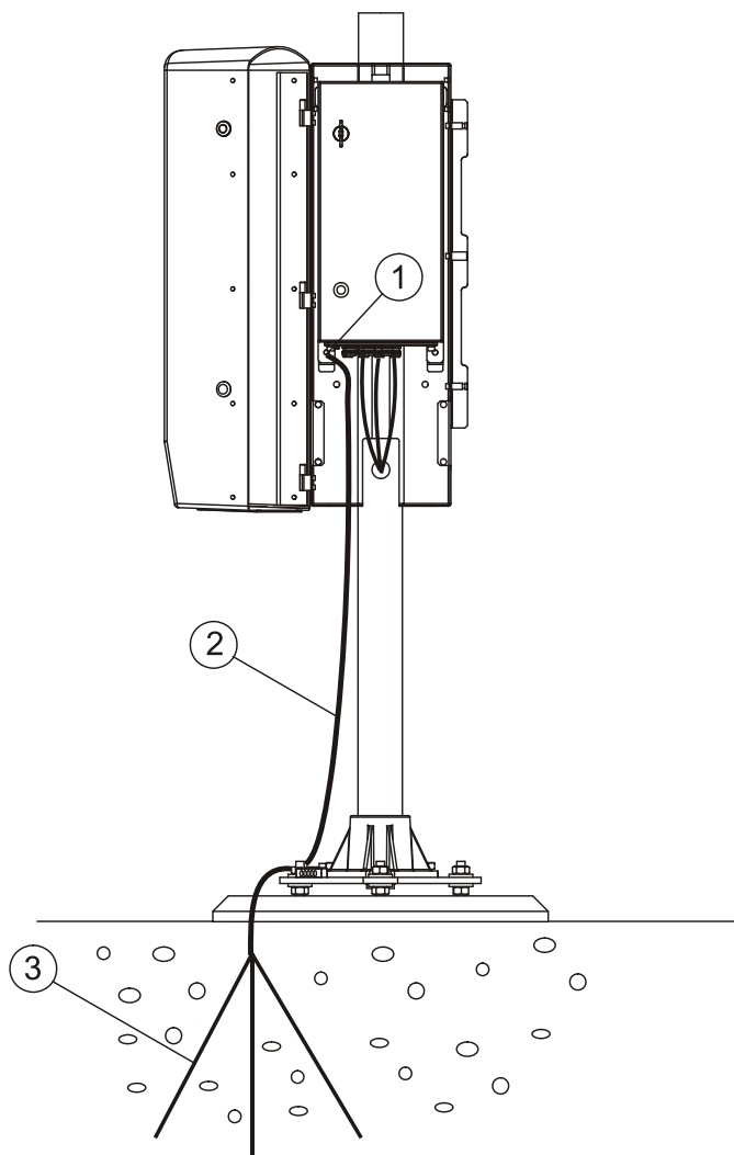
Рис. 3. Заземление оборудования FS11P
