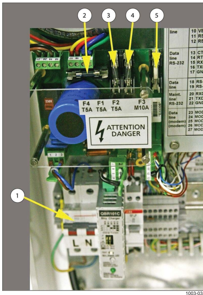
Рис. 50. Расположение предохранителей на плате FSP103.
