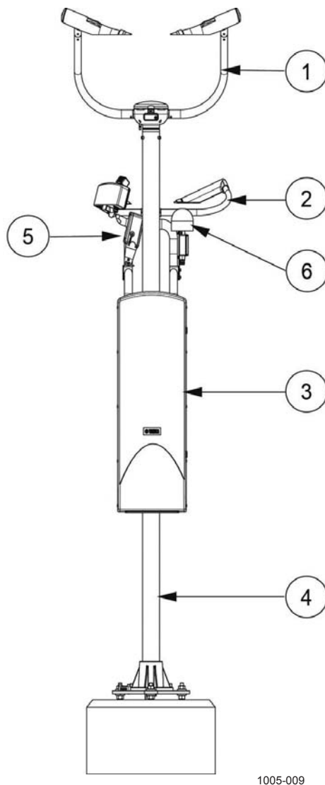
Рис. 1. Система FS11P
