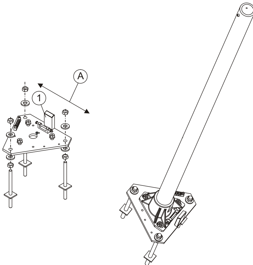
Рис. 8. Установка мачты FS11P с помощью монтажного комплекта FS211296
