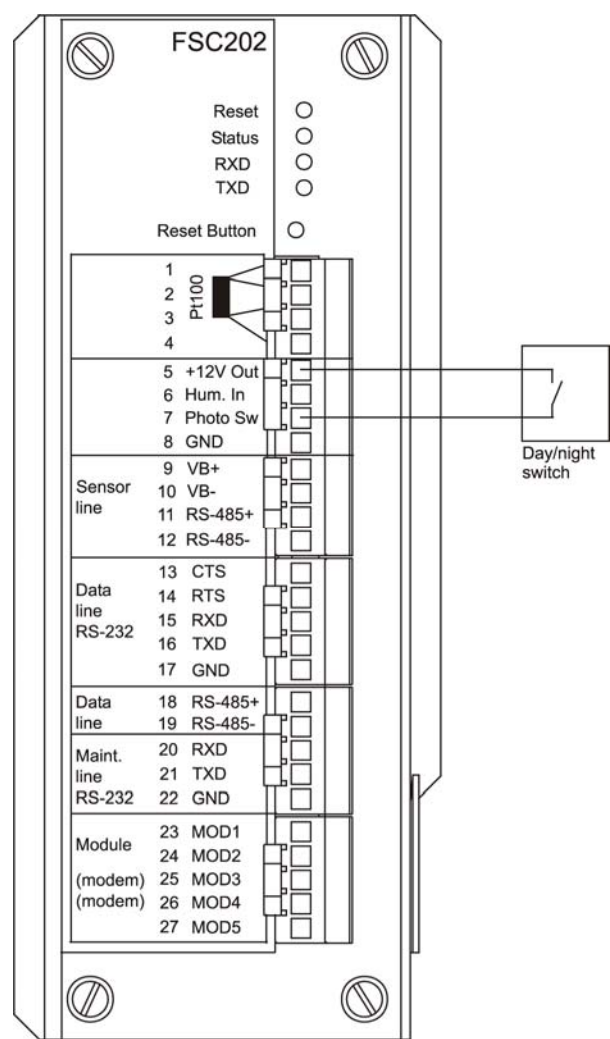
Рис. 32. Подключение фотопереклюателя день/ночь
