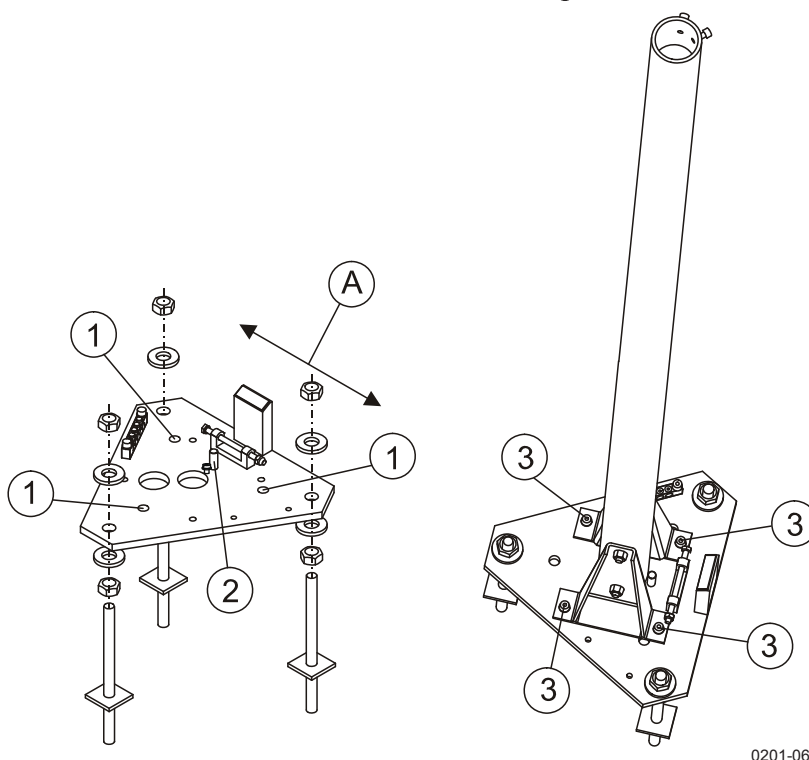
Рис. 10. Установка алюминиевой мачты FS11P с помощью монтажного комплекта FS211296
