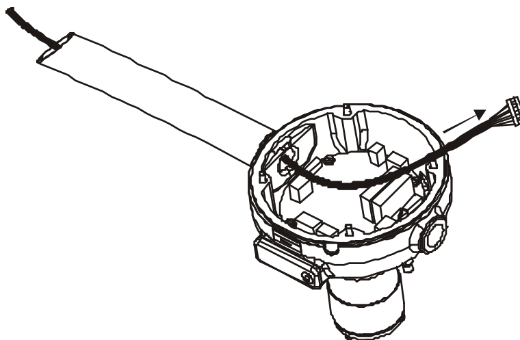
Рис. 47. Вытягивание контрольного кабеля из трубы корпуса
