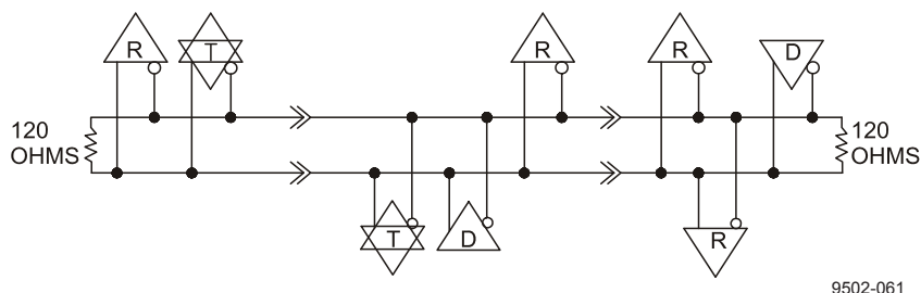
Рис. 28. Применение RS-485
