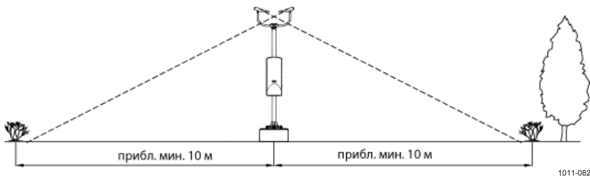
Рис. 2. Рекомендуемое расположение датчика текущей погоды FS11P с мачтой FSAM250/FSFM250
