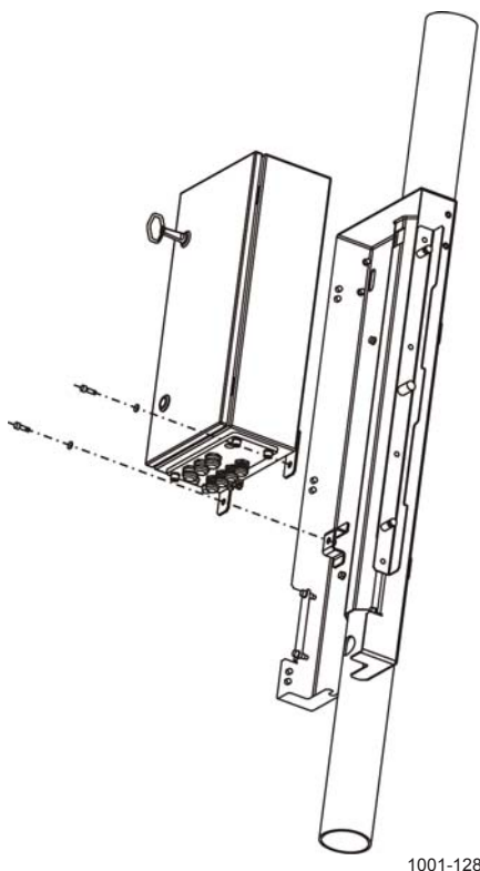
Рис. 19. Установка корпуса интерфейсного блока
