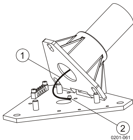
Рис. 9. Монтаж кабеля заземления хрупкой мачты FS11P
